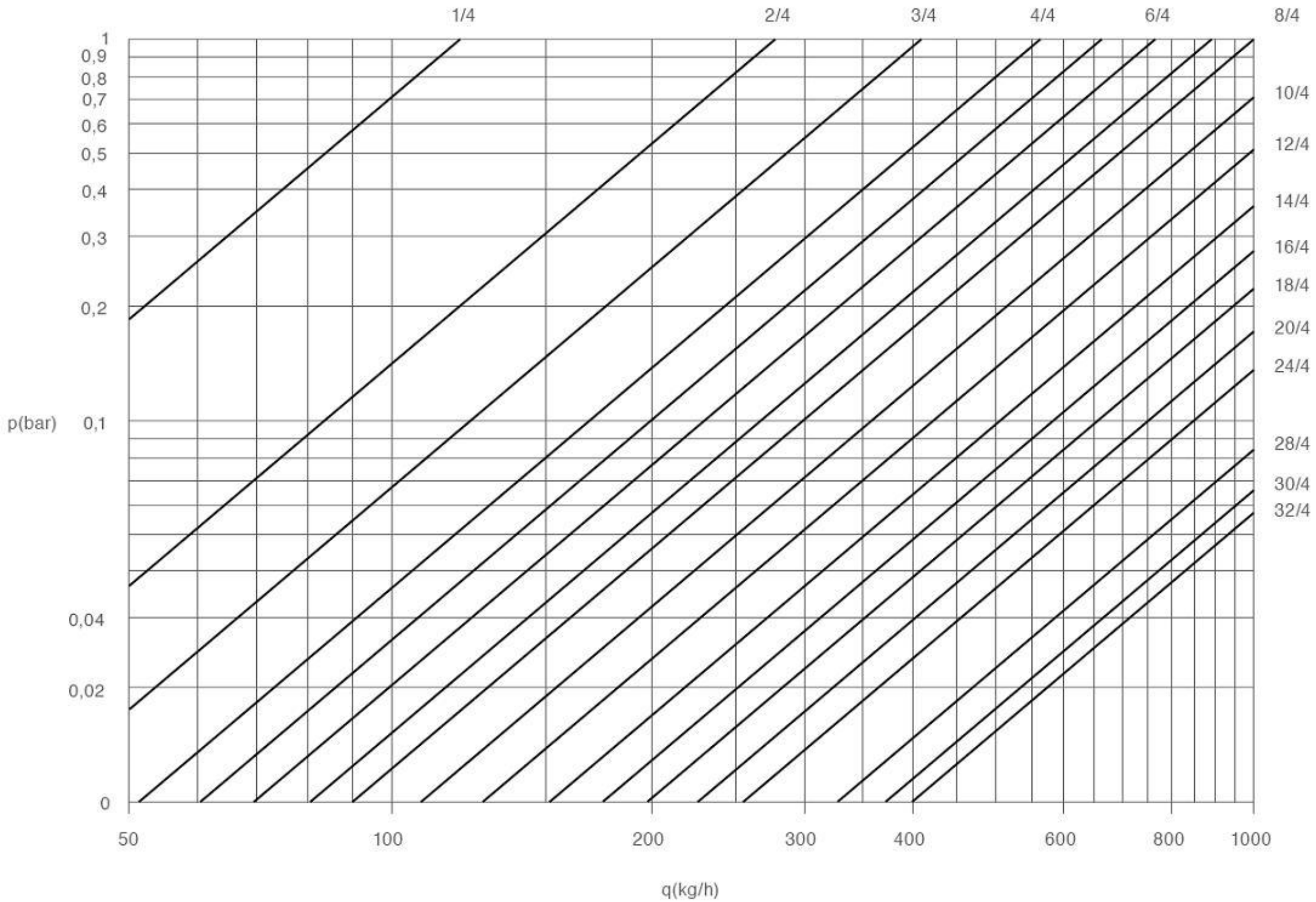
G 3/4"-os és G 1"-os osztó-gyűjtők fojtási diagramja (1/4 fordulatonként)
